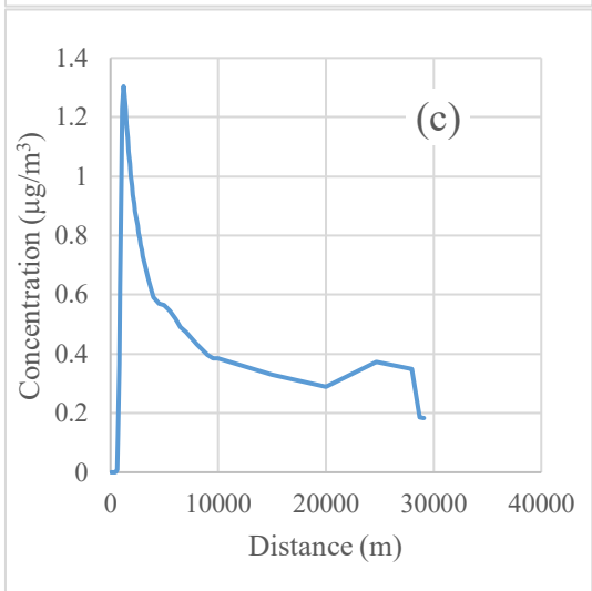
شکل ۴- حداکثر غلظت آلاینده‌ها بر حسب فاصله از دودکش در جهت جنوب‌شرقی: (a) SO 2 , (b) NO 2 و (c) CO
