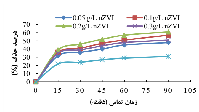
شکل ۴: تاثیر تغییرات دز نانو ذرات آهن صفر در راندمان حذف آنتی بیوتیک تتراسایکلین در شرایط آزمایش (غلظت اولیه آنتی بیوتیک (۱۵mg/L)، pH (۷)، توان لامپ UV ۸ وات)؛ زمان تماس متغیر
