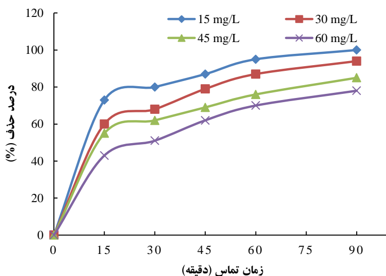
شکل ۸: تاثیر تغییرات غلظت آنتی بیوتیک تتراسایکلین بر کارایی فرآیند UV/H 2 O 2 /nZVI در شرایط بهینه آزمایش (H 2 O 2 = ۸۰ mmol/L ، pH=۳ ، nZVI=۰/۲ g/L ، UV=۵۰ وات؛ زمان تماس متغیر
