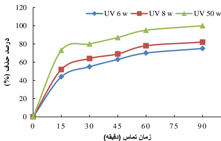
شکل ۷: تاثیر تغییرات توان لامپ UV بر راندمان حذف آنتی بیوتیک تتراسایکلین در شرایط بهینه آزمایش (H 2 O 2 = 80 mmol/L، nZVI= 0/2 g/L، pH= ۳) و غلظت اولیه آنتی بیوتیک تتراسایکلین (15 mg/L)؛ زمان تماس متغیر
