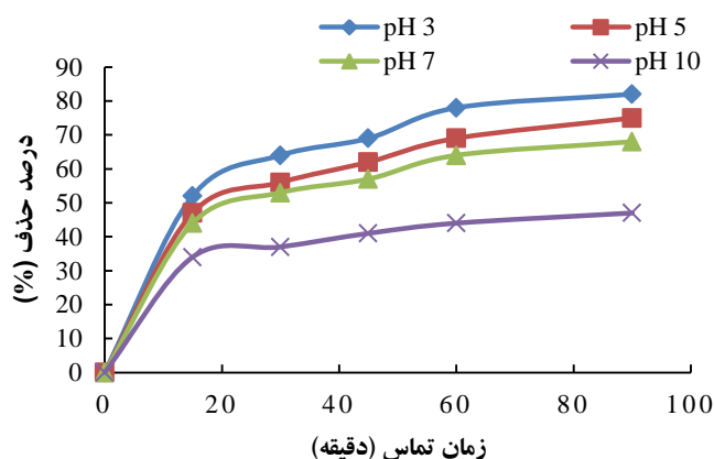
نمودار ۶: تاثیر تغییرات pH بر راندمان حذف آنتی بیوتیک تتراسایکلین در شرایط آزمایش: غلظت اولیه آنتی بیوتیک تتراسایکلین (15 mg/L)، توان لامپ UV (۸ وات)، غلظت بهینه پراکسید هیدروژن (80 mmol/L) و دز نانو ذره آهن صفر (بهینه 0/2 g/L)؛ زمان تماس متغیر
