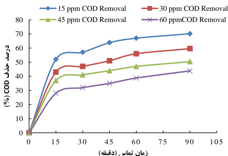
شکل ۸. مقایسه میزان حذف آنتی بیوتیک تتراسایکلین و COD فاضلاب در شرایط بهینه فرآیند تلفیقی UV/H 2 O 2 /nZVI در غلظت های ۱۵-۳۰-۴۵-۶۰ mg/L آنتی بیوتیک تتراسایکلین
