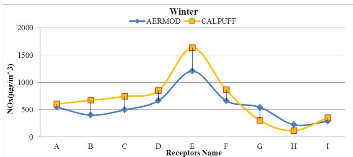
شکل ۶. مقایسه نتایج حاصل از اجرای دو مدل AERMOD و CALPUFF در ۹ ایستگاه پذیرنده فصل زمستان
