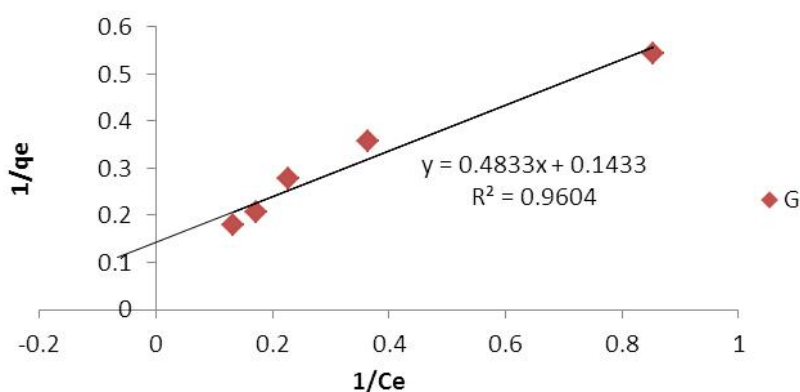
نمودار ۷: ایزوترم لانگمویر در حذف فلوراید توسط G
