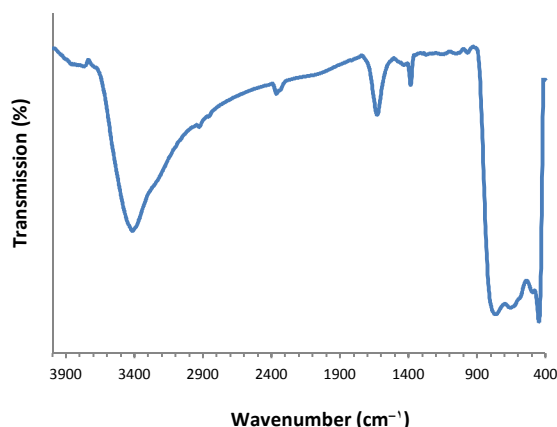
شکل ۳: طیف FTIR نانو ذرات TiO_2
