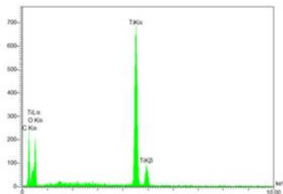
شکل ۴: طیف EDX فوتوکاتالیزور TiO_2
