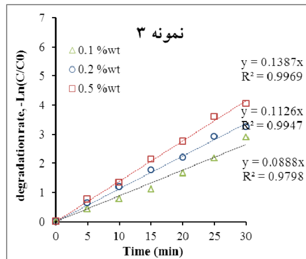
شکل ۹: تغییرات سرعت تجزیه فتوکاتالیستی متیل اورانژ نسبت به زمان با استفاده از نمونه ۳
