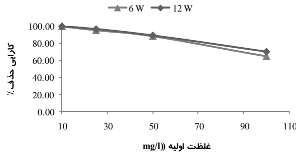
نمودار ۴: تأثیر غلظت اولیه سفالکسین برای توان 6 وات و 12 وات (pH=3, دوز نانو ذره برابر 0.1 گرم در لیتر و زمان تماس 15 دقیقه برای توان 12 وات و زمان تماس 30 دقیقه برای توان 6 وات)
