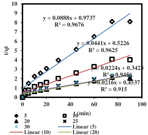
نمودار ۱۰: نمودار سینتیک شبه درجه اول و شبه درجه دوم جذب آلاینده تتراسایکلین توسط جاذب کیتوزان مغناطیسی شده بی متالیک
