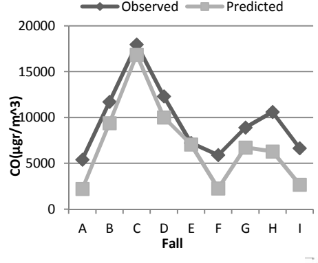
شکل ۳: مقایسه مقادیر شبیه‌سازی و پای‌CO در ۹ ایستگاه پذیرنده
