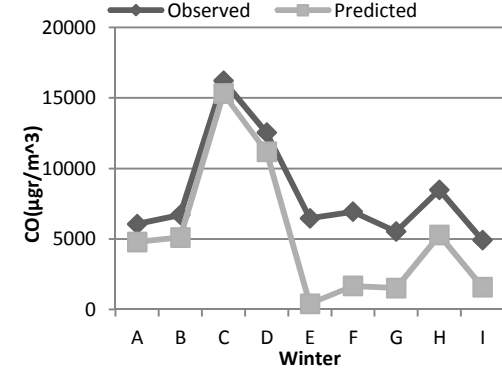
شکل ۳: مقایسه مقادیر شبیه‌سازی و پای‌CO در ۹ ایستگاه پذیرنده
