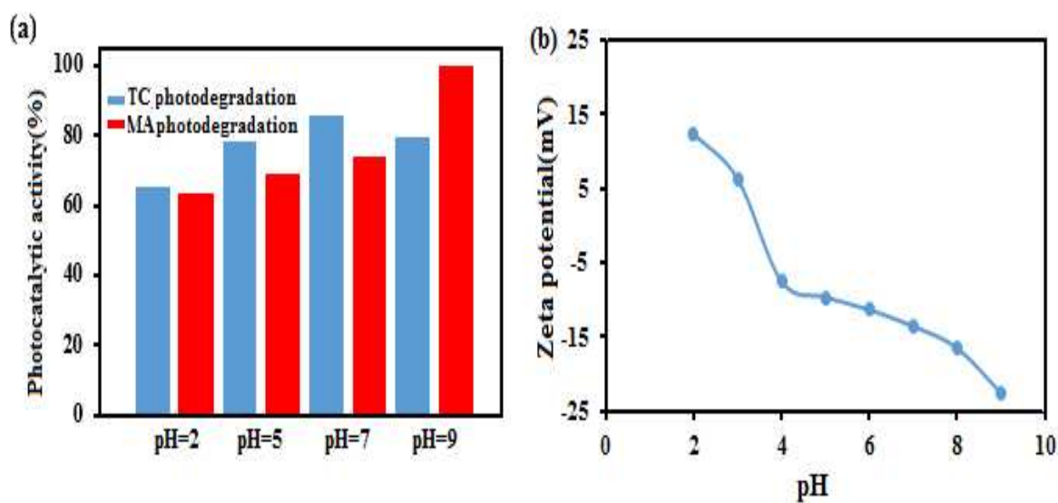
شکل ۵. تخریب فوتوکاتالیستی آلایند تتراسایکلین و مالاتیون در pH های مختلف (a)، نمودار PZC (b)
