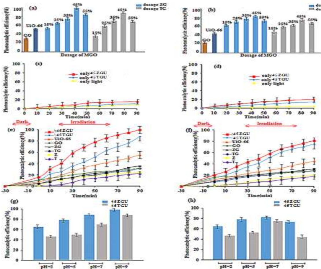
شکل ۱. نمودار درصد تخریب آلایند (a) مالاتیون و (b) تتراسایکلین با نسبت های جرمی مختلف؛ وابستگی درصد حذف آلایند (c) مالاتیون و (d) تتراسایکلین به حضور نور و فوتوکاتالیست؛ نمودار درصد تخریب آلایند (e) مالاتیون و (f) تتراسایکلین در حضور فوتوکاتالیست های مختلف؛ نمودار درصد تخریب آلایند (g) مالاتیون و (h) تتراسایکلین در pH های مختلف
