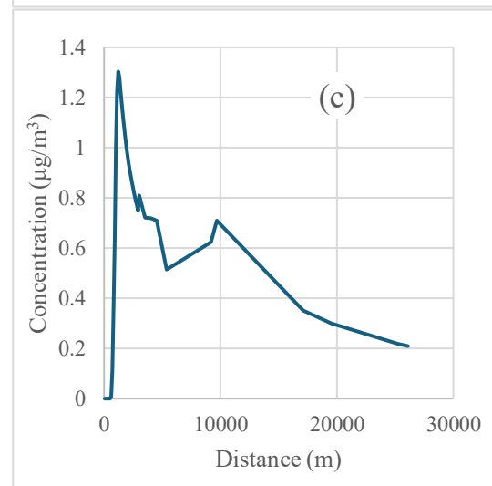
شکل ۷. حداکثر غلظت آلاینده‌ها بر حسب فاصله از دودکش در جهت شمال \text{SO}_2 (a)، \text{NO}_2 (b) و \text{CO} (c)
