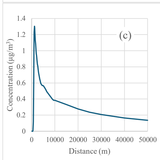
شکل ۳. حداکثر غلظت آلاینده‌ها بر حسب فاصله از دودکش در جهت‌های غرب، جنوب غربی و جنوب: \text{SO}_2 (a)، \text{NO}_2 (b) و \text{CO} (c)
