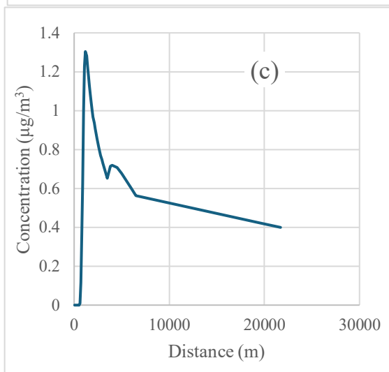
شکل ۸. حداکثر غلظت آلاینده‌ها بر حسب فاصله از دودکش در جهت شمال غربی \text{SO}_2 (a)، \text{NO}_2 (b) و \text{CO} (c)
