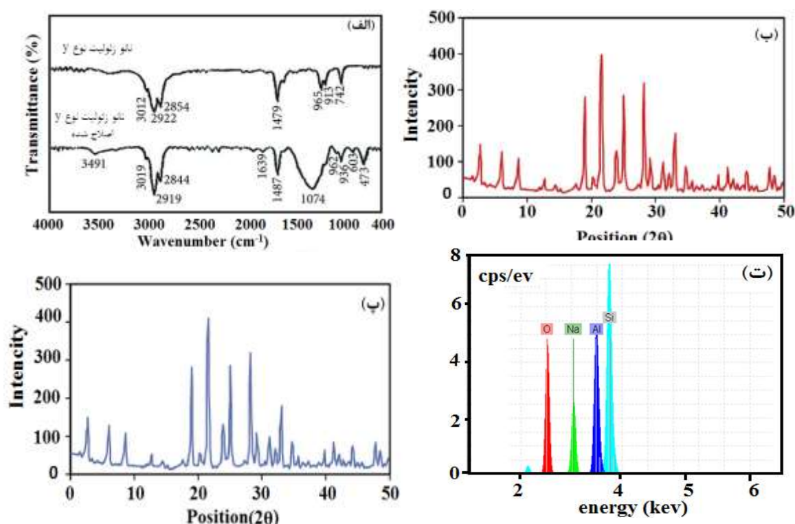
شکل ۱: (الف) تصویر FTIR از نانو ژئولیت نوع \gamma قبل و بعد از اصلاح (ب) تصویر XRD برای نانو ژئولیت نوع \gamma (پ) تصویر XRD نانو ژئولیت نوع \gamma اصلاح شده (ت) تصویر EDX از نانو ژئولیت نوع \gamma
