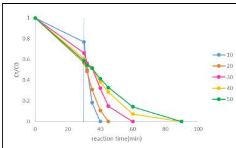
نمودار ۶: تأثیر غلظت آلاینده بر تجزیه سفیکسیم در فرآیند فتوکاتالیستی (۶-۷، pH = ۶،۵، ۲mM، PS = دوز فتوکاتالیست = ۰،۱ g/L)
