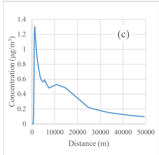
شکل ۵- حداکثر غلظت آلاینده‌ها بر حسب فاصله از دودکش در جهت شرق (a) \text{SO}_2 ، (b) \text{NO}_2 و (c) \text{CO}
