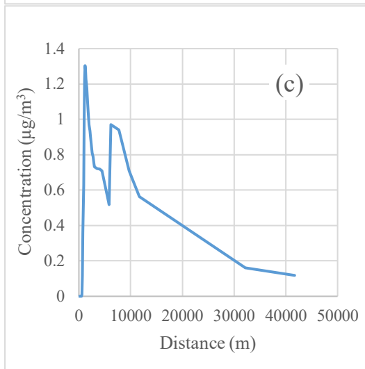
شکل ۶- حداکثر غلظت آلاینده‌ها بر حسب فاصله از دودکش در جهت شمال شرقی (a) \text{SO}_2 ، (b) \text{NO}_2 و (c) \text{CO}
