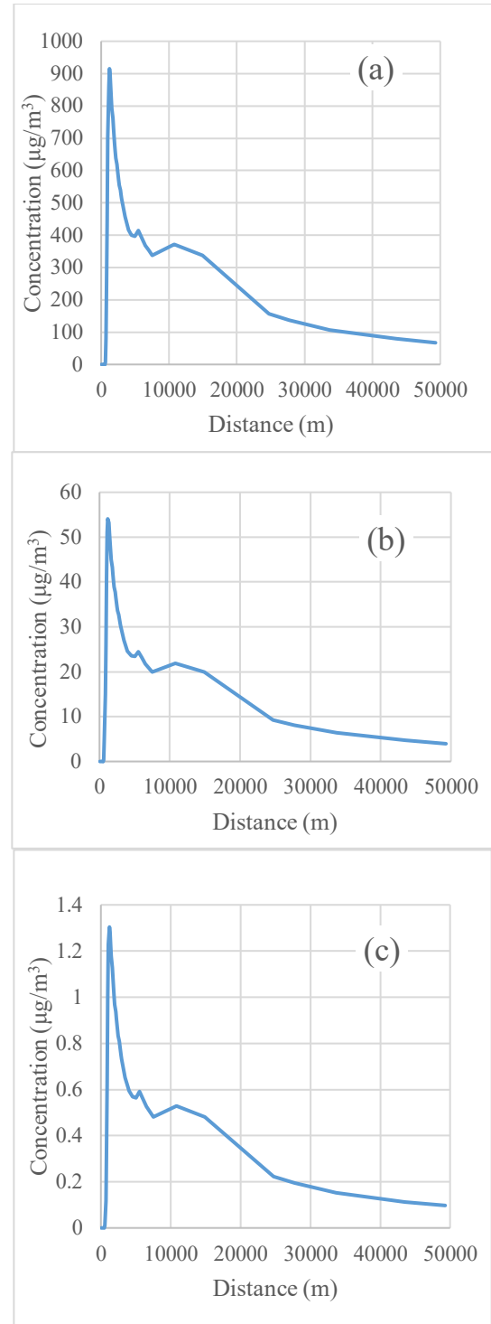
شکل ۵- حداکثر غلظت آلاینده‌ها بر حسب فاصله از دودکش در جهت شرق (a) \text{SO}_2 ، (b) \text{NO}_2 و (c) \text{CO}
