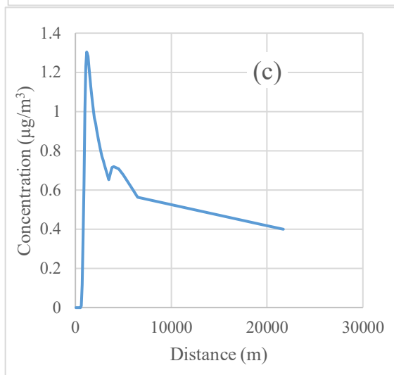
شکل ۸- حداکثر غلظت آلاینده‌ها بر حسب فاصله از دودکش در جهت شمال غربی (a) \text{SO}_2 ، (b) \text{NO}_2 و (c) CO
