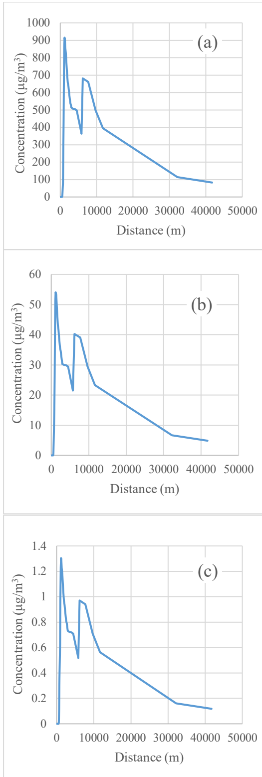
شکل ۶- حداکثر غلظت آلاینده‌ها بر حسب فاصله از دودکش در جهت شمال‌شرقی (a) \text{SO}_2 ، (b) \text{NO}_2 و (c) \text{CO}
