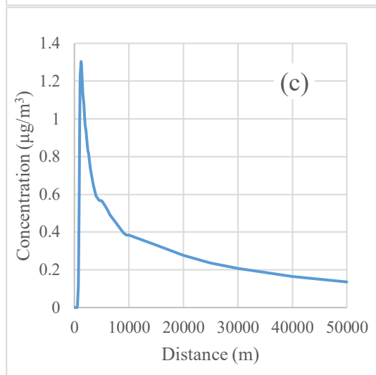
شکل ۳- حداکثر غلظت آلاینده‌ها بر حسب فاصله از دودکش در جهت‌های غرب، جنوب غربی و جنوب: (a) \text{SO}_2 , (b) \text{NO}_2 و (c) \text{CO}
