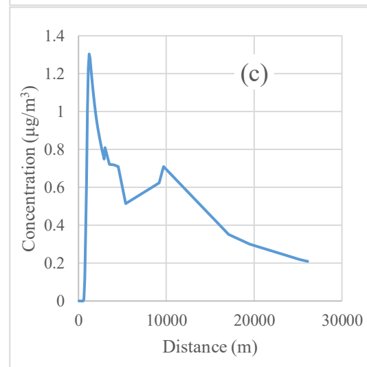
شکل ۷- حداکثر غلظت آلاینده‌ها بر حسب فاصله از دودکش در جهت شمال (a) \text{SO}_2 ، (b) \text{NO}_2 و (c) CO
