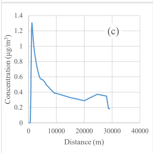
شکل ۴- حداکثر غلظت آلاینده‌ها بر حسب فاصله از دودکش در جهت جنوب شرقی: (a) \text{SO}_2 , (b) \text{NO}_2 و (c) \text{CO}
