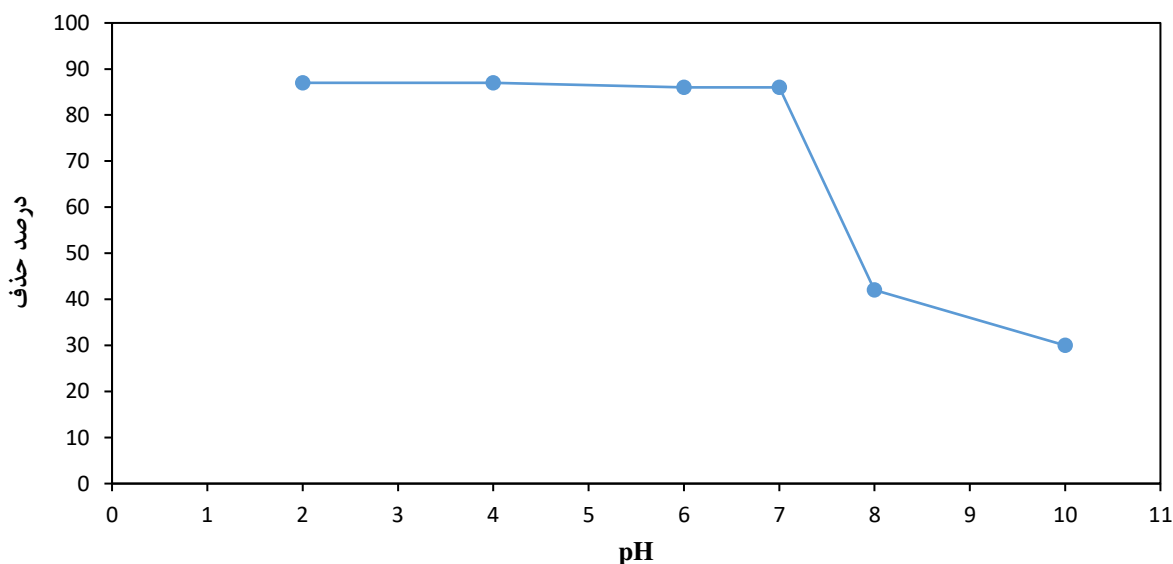
شکل ۱. اثر pH محلول بر راندمان حذف مالاتیون توسط کربن فعال در شرایط: دوز جاذب ۱ g/L، غلظت اولیه مالاتیون ۵۰ mg/L، زمان تماس ۱۵ دقیقه و دمای محیط
