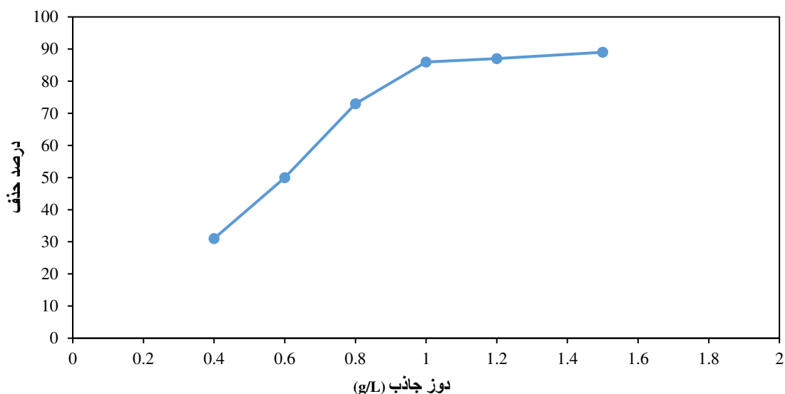
شکل ۲. اثر دوز جاذب بر درصد حذف مالاتیون توسط کربن فعال در شرایط \text{pH}=7 غلظت اولیه مالاتیون 50 \text{ mg/L} ، زمان تماس ۱۵ دقیقه و دمای محیط
