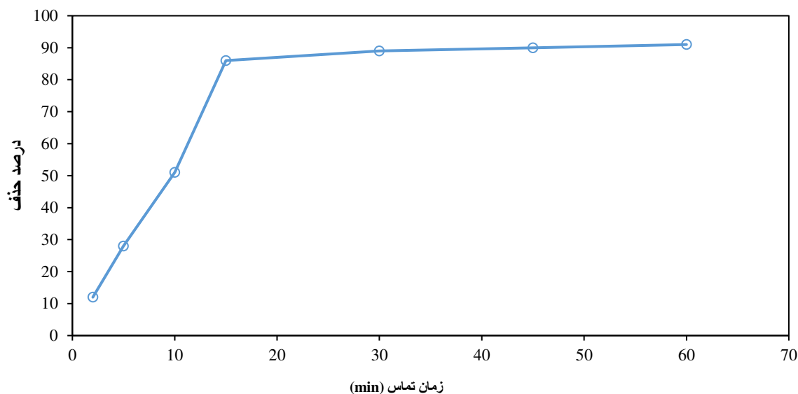
شکل ۳. اثر زمان تماس بر راندمان حذف مالاتیون توسط کربن فعال در شرایط \text{pH}=7 ، دوز جاذب 1 \text{ g/L} ، غلظت اولیه مالاتیون 50 \text{ ppm} و دمای محیط
