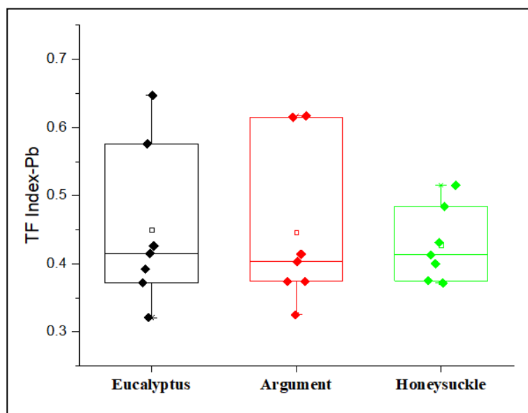
شکل ۶. مقایسه مقادیر شاخص تجمع زیستی فلز سنگین سرب در برگ درختان اوکالپتوس، برهان و کهور در سطح شهر اهواز
