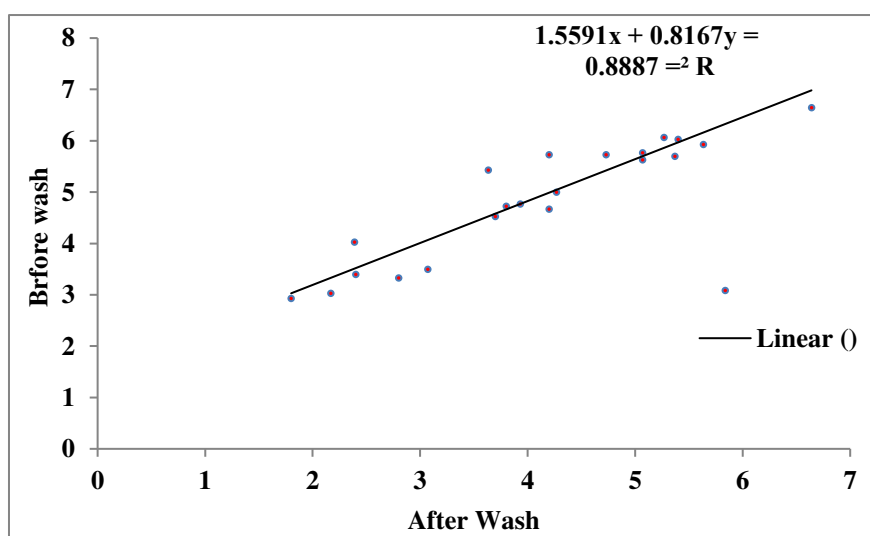
شکل ۷. برازش رگرسیونی مقادیر سرب برگ‌های شسته نشده و شسته شده درختان اوکالپتوس، برهان و کهور سطح شهر اهواز
