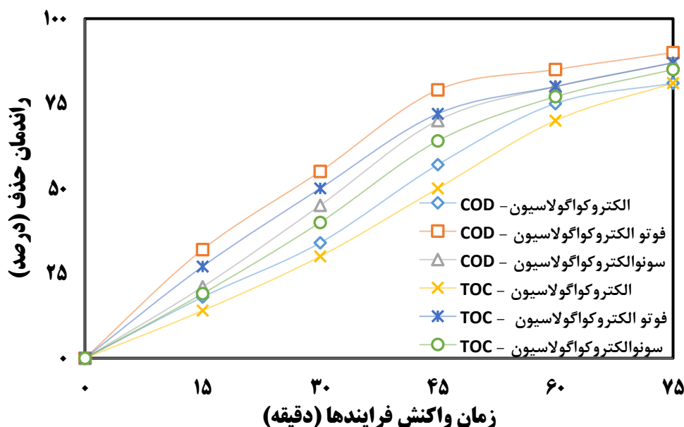
شکل ۶. نتایج حذف COD و TOC میکروپلاستیک پلی اتیلن در شرایط بهینه ( pH=9/6 ، جریان الکتریکی = ۳ آمپر، فاصله بین الکترودها = ۱ سانتی متر، تعداد الکترودها = ۶ عدد، غلظت میکروپلاستیک پلی اتیلن = ۵۰ میلی گرم در لیتر و زمان واکنش = ۷۵ دقیقه)
