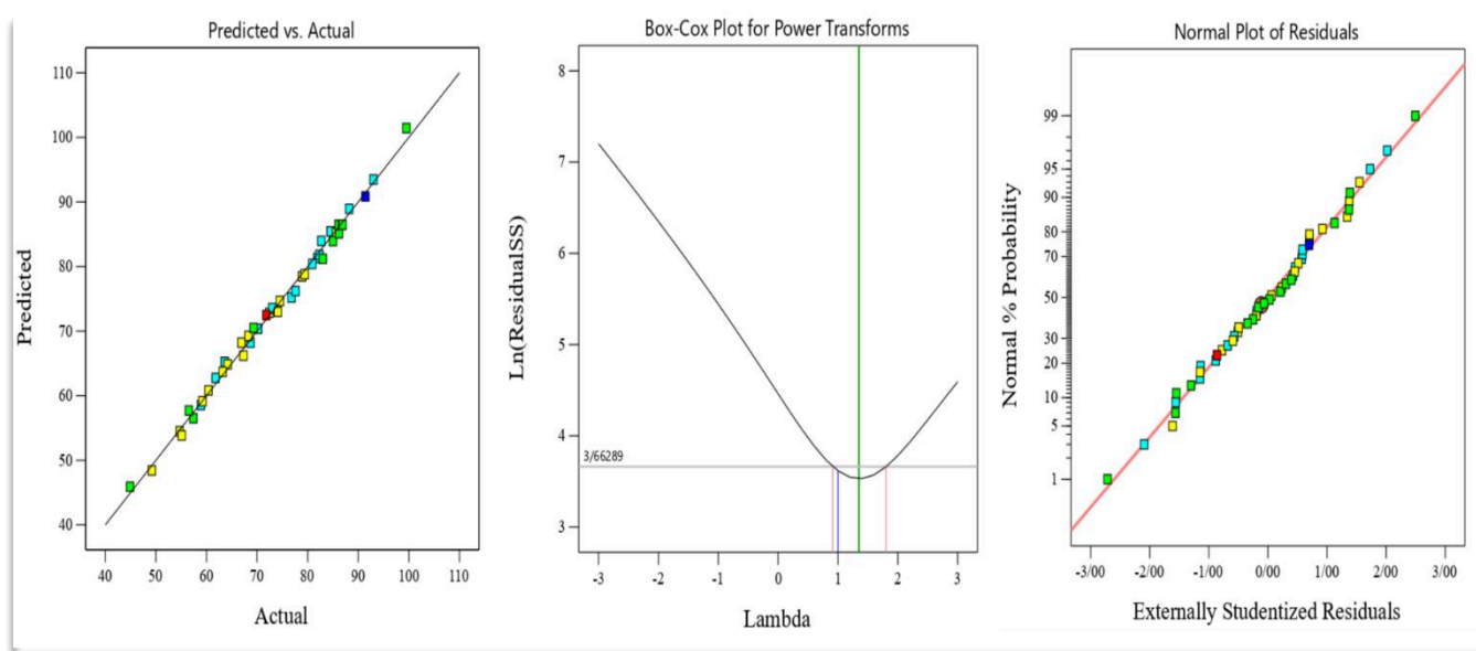
شکل ۲. نمودارهای تشخیصی مدل درجه دوم راندمان حذف میکروپلاستیک پلی اتیلن در فرایند الکتروکواگولاسیون
