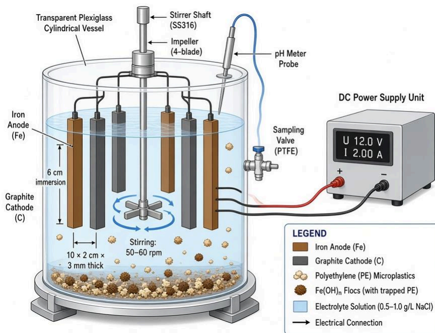
شکل ۱. شماتیک پایلوت فرایند الکتروکواگولاسیون در حذف میکروپلاستیک پلی اتیلن
