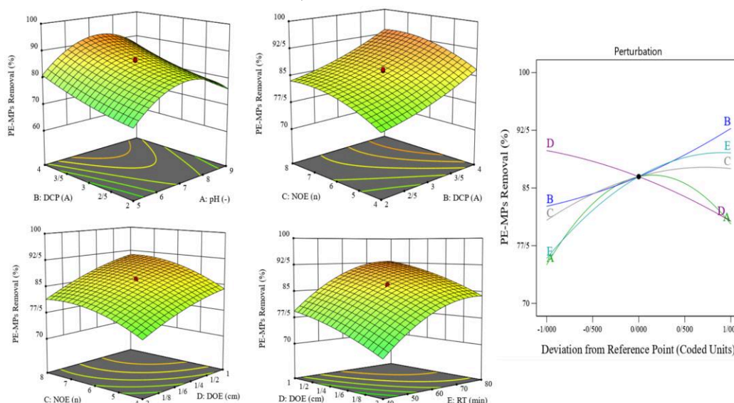
شکل ۳. نمودارهای سه بعدی سطح پاسخ و نمودار اغتشاش اثرات متقابل متغیرهای عملیاتی بر راندمان حذف میکروپلاستیک پلی اتیلن
