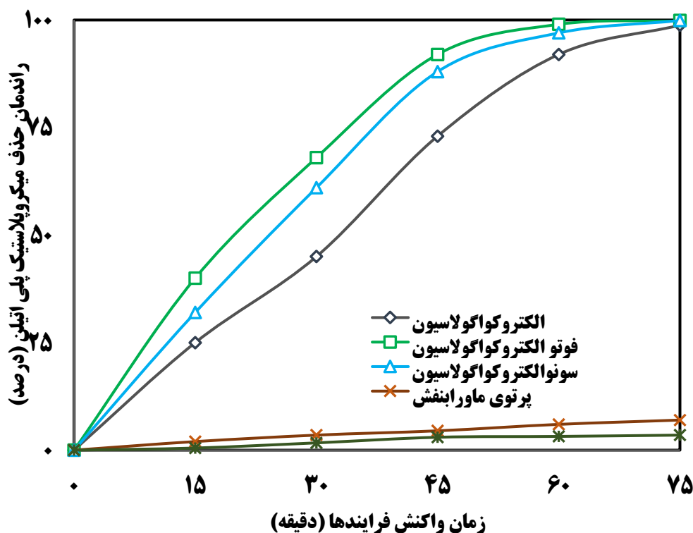
شکل ۵. مقایسه حذف میکروپلاستیک پلی اتیلن در سیستم‌های متفاوت در شرایط بهینه ( \text{pH}=9/6 ، جریان الکتریکی = ۳ آمپر، فاصله بین الکترودها = ۱ سانتی‌متر، تعداد الکترودها = ۶ عدد، غلظت میکروپلاستیک پلی اتیلن = ۵۰ میلی گرم در لیتر و زمان واکنش = ۷۵ دقیقه)
