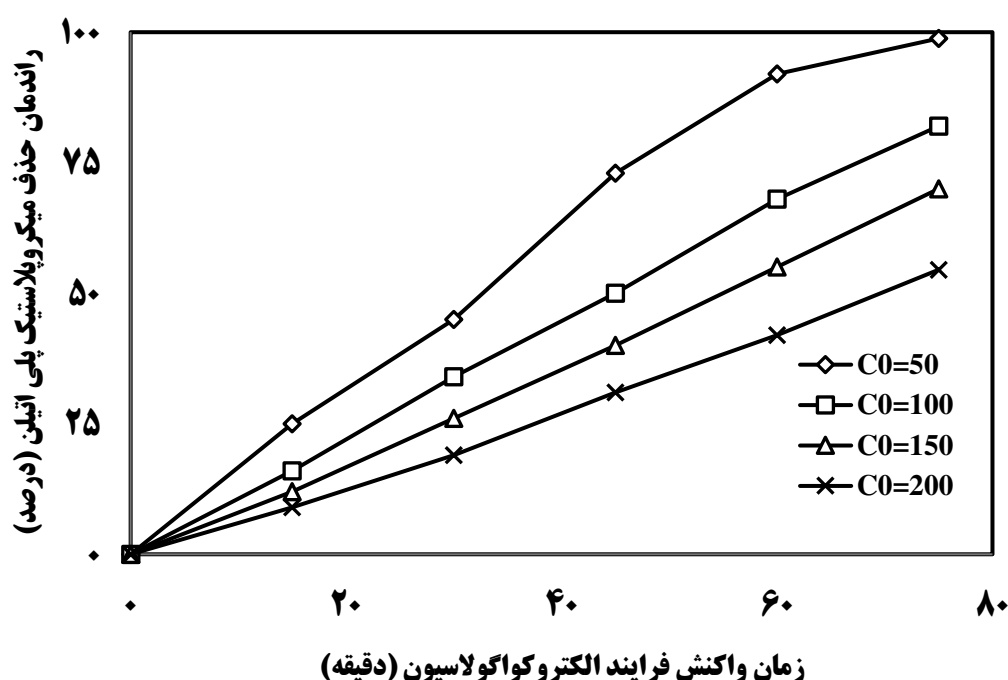
شکل ۴. اثر غلظت اولیه میکروپلاستیک پلی اتیلن بر راندمان فرایند الکتروکواگولاسیون در شرایط بهینه ( \text{pH}=6/9 ، جریان الکتریکی = ۳ آمپر، فاصله بین الکترودها = ۱ سانتی‌متر، تعداد الکترودها = ۶ عدد و زمان واکنش = ۷۵ دقیقه)
