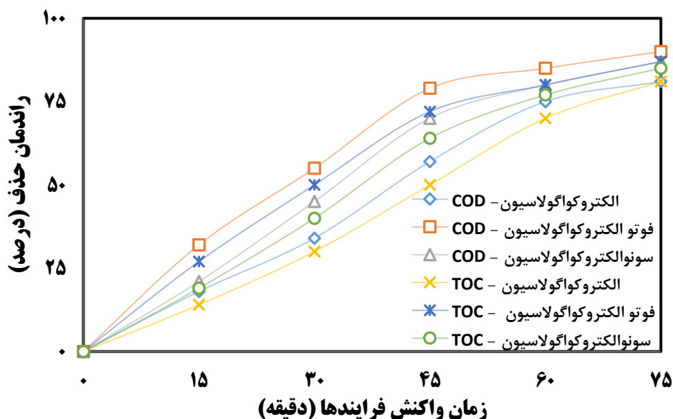
شکل ۶. نتایج حذف COD و TOC میکروپلاستیک پلی اتیلن در شرایط بهینه (pH=۹/۶، جریان الکتریکی = ۳ آمپر، فاصله بین الکترودها = ۱ سانتی متر، تعداد الکترودها = ۶ عدد، غلظت میکروپلاستیک پلی اتیلن = ۵۰ میلی گرم در لیتر و زمان واکنش = ۷۵ دقیقه)
