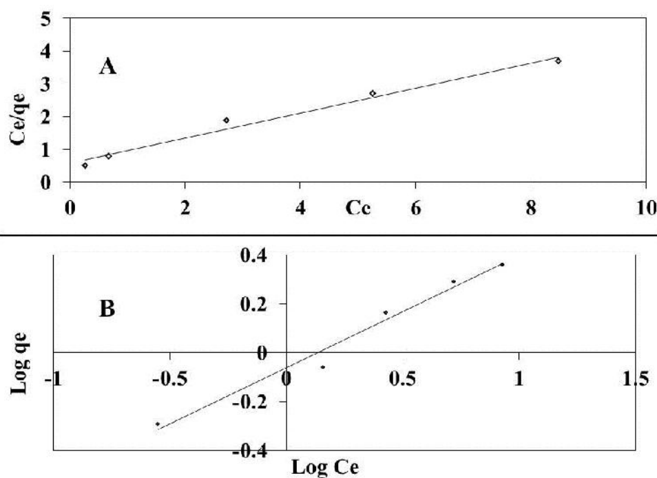
شکل ۱۰: نتایج بررسی مدل‌های ایزوترمی (a) لانگمویر و (b) فروندلیخ (دوز جاذب: ۵ g/L، غلظت فلوراید: ۱۵-۳-۶ mg/L، pH=۶)
