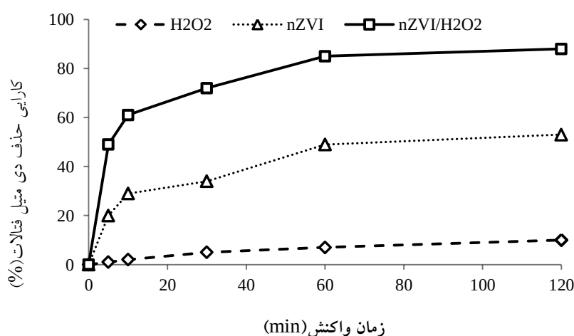
شکل ۵: تأثیر nZVI.H_2O_2 و nZVI/H_2O_2 در حذف دی‌متیل‌فتالات
