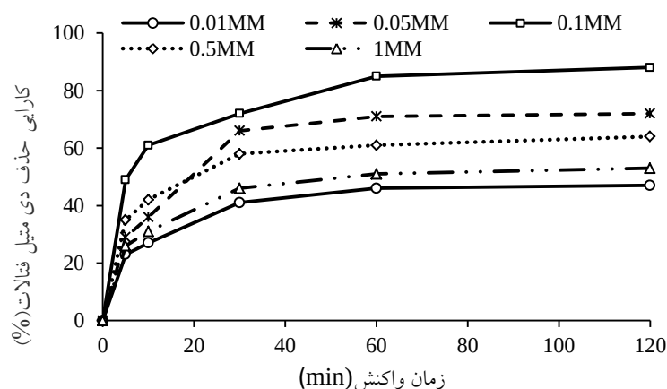
شکل ۲: تأثیر غلظت پراکسید هیدروژن در حذف دی‌متیل فتالات
