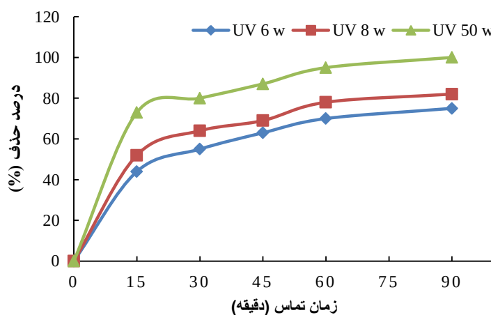
شکل ۷: تاثیر تغییرات توان لامپ UV بر راندمان حذف آنتی بیوتیک تتراسایکلین در شرایط بهینه آزمایش ( 80 \text{ mmol/L} \text{H}_2\text{O}_2 ، \text{nZVI} = 0.2 \text{ g/L} ، \text{pH} = 3 ) و غلظت اولیه آنتی بیوتیک تتراسایکلین ( 15 \text{ mg/L} )؛ زمان تماس متغیر
