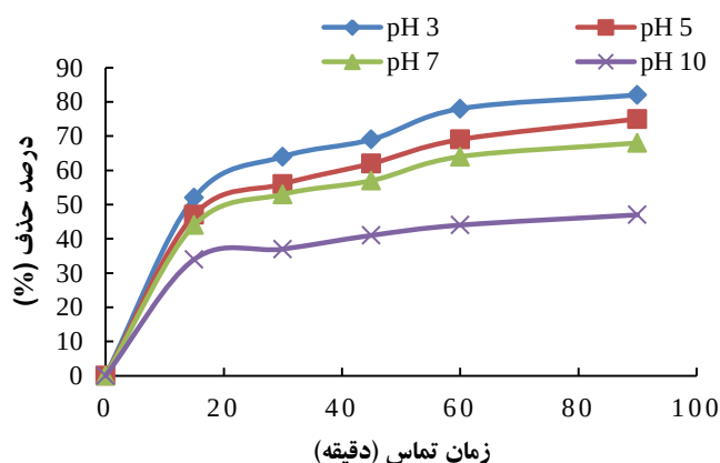
نمودار ۶: تاثیر تغییرات pH بر راندمان حذف آنتی بیوتیک تتراسایکلین در شرایط آزمایش: غلظت اولیه آنتی بیوتیک تتراسایکلین ( 15 \text{ mg/L} )، توان لامپ UV (۸ وات)، غلظت بهینه پراکسید هیدروژن ( 80 \text{ mmol/L} ) و دز نانو ذره آهن صفر (بهینه 0.2 \text{ g/L} )؛ زمان تماس متغیر
