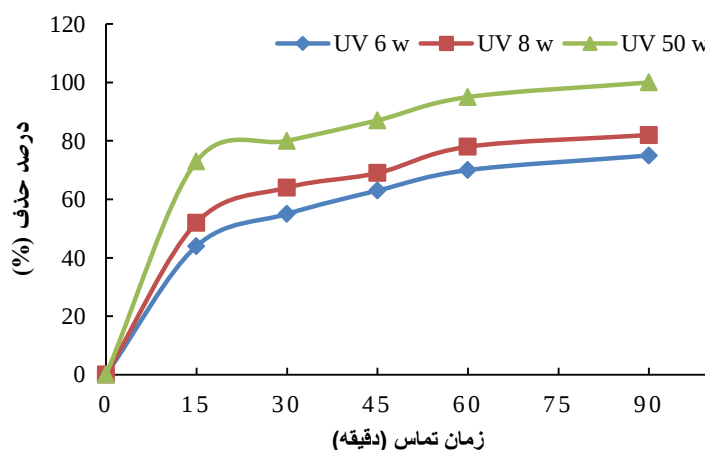
شکل ۷: تاثیر تغییرات توان لامپ UV بر راندمان حذف آنتی بیوتیک تتراسایکلین در شرایط بهینه آزمایش (۸۰ mmol/L H 2 O 2 ، nZVI= ۰/۲ g/L، pH= ۳) و غلظت اولیه آنتی بیوتیک تتراسایکلین (۱۵ mg/L)؛ زمان تماس متغیر
