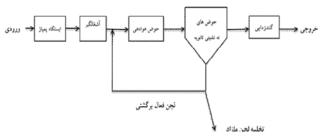
شکل ۱: فلودیگرام فرایند لجن فعال هوادهی گسترده تصفیه خانه فاضلاب بیمارستان گلستان اهواز
