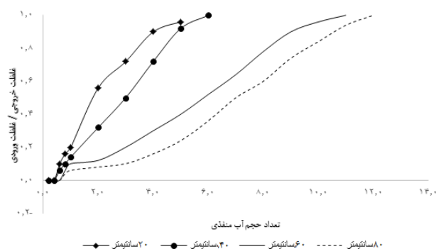
شکل ۶: منحنی رخنه مربوط به ضخامت های مختلف خاک
