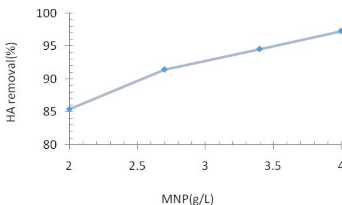
شکل ۴: اثر تغییرات دوز نانو ذرات مغناطیسی بر راندمان حذف هیومیک اسید (غلظت هیومیک اسید 10 mg/L، زمان تماس ۹۰ دقیقه، pH برابر با ۴/۵، دما ۲۵ درجه سانتیگراد، شدت اختلاط ۲۵۰ rpm)
