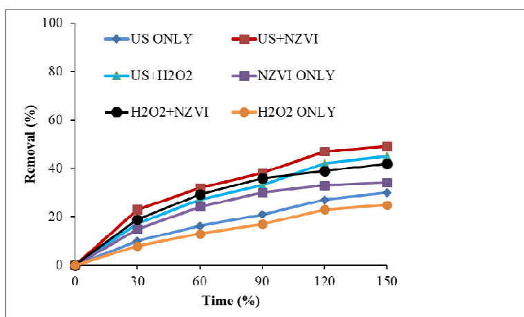
شکل ۶: تأثیر عوامل حذف در غیاب یک یا دو عامل (در شرایط \text{AMX}=45 \text{ ppm} ، \text{pH}=3 ، \text{H}_2\text{O}_2=0.3\% ، \text{nZVI}=0.2 \text{ g/L} و فرکانس ۱۳۰ کیلوهرتز)
