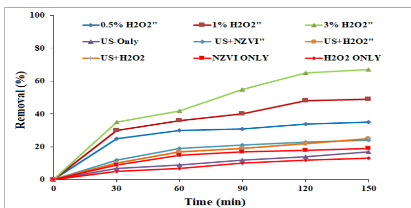
شکل ۷: کارایی سیستم در حذف COD (در شرایط \text{AMX}=45 \text{ ppm} ، \text{pH}=3 ، \text{H}_2\text{O}_2=0.3\% ، \text{nZVI}=0.2 \text{ g/L} و فرکانس ۱۳۰ کیلوهرتز)
