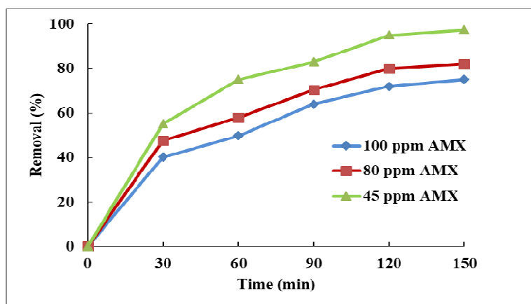
شکل ۵: تأثیر غلظت اولیه آنتی بیوتیک آموکسی سیلین بر کارایی سیستم (در شرایط \text{pH}=3 ، \text{H}_2\text{O}_2=0.3\% ، \text{nZVI}=0.2 \text{ g/L} و فرکانس ۱۳۰ کیلوهرتز)
