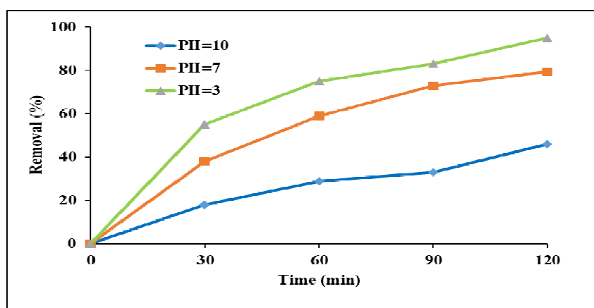
شکل ۳: تأثیر pH بر کارایی حذف آنتی‌بیوتیک آموکسی سیلین (در شرایط nZVI = 0.2 \text{ g/L} ، AMX = 45 \text{ ppm} و H_2O_2 = 3\% و فرکانس ۱۳۰ کیلوهرتز)
