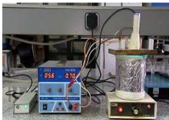
شکل ۱: تصویر شماتیک و واقعی راکتور مورد استفاده
