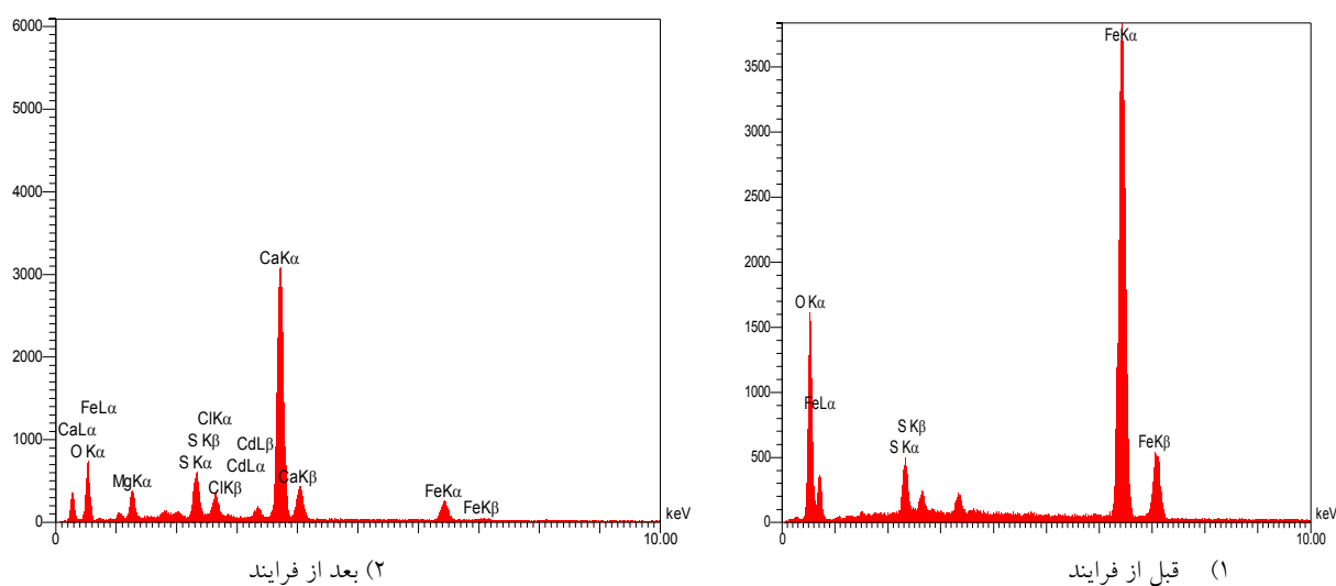
تصویر ۵: نتایج مربوط به تصویر برداری SEM و گراف مربوط به EDAX نمونه لجن قبل و بعد از فرایند
