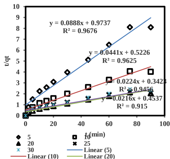
نمودار ۱۰: نمودار سینتیک شبه درجه اول و شبه درجه دوم جذب آلاینده تتراسایکلین توسط جاذب کیتوزان مغناطیسی شده بی متالیک
