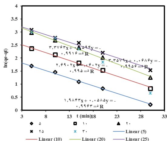
نمودار ۱۰: نمودار سینتیک شبه درجه اول و شبه درجه دوم جاذب آلاینده تتراسایکلین توسط کیتوزان مغناطیسی شده بی متالیک
