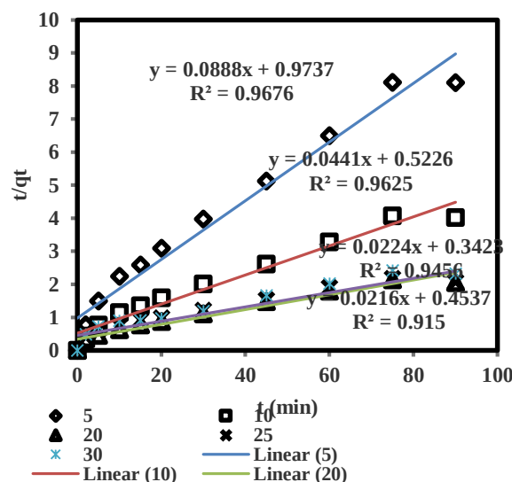
نمودار ۱۰: نمودار سینتیک شبه درجه اول و شبه درجه دوم جاذب آلاینده تتراسایکلین توسط کیتوزان مغناطیسی شده بی متالیک
