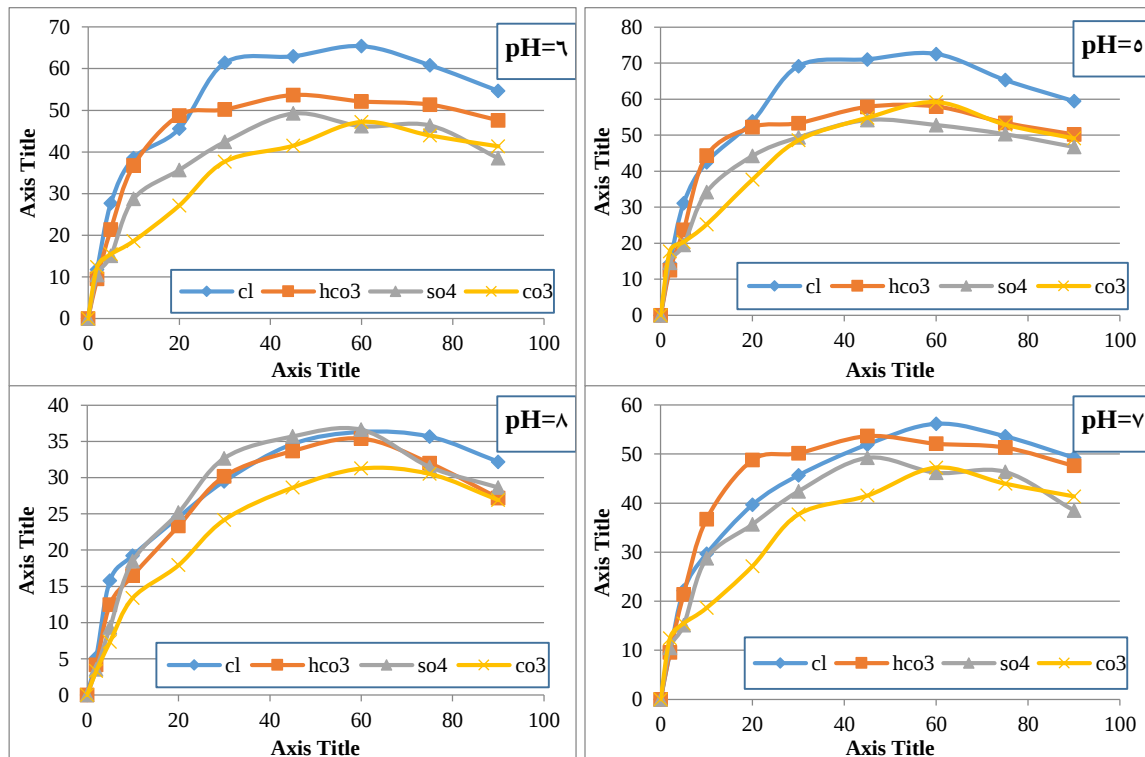
شکل ۵: تأثیر تغییر pH بر راندمان حذف آنیون‌های مزاحم توسط نانو کامپوزیت کیتوزان مغناطیسی شده بی متالیک
