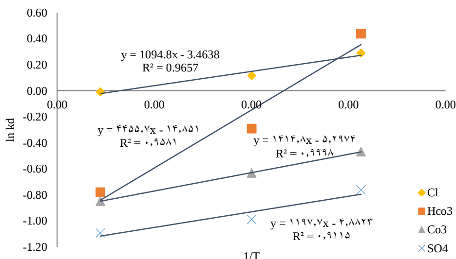
شکل ۱۳-۱: نمودار ترمودینامیک جذب آنیون‌های مزاحم (کلراید، سولفات، کربنات و بی‌کربنات) توسط جاذب کیتوزان مغناطیسی شده بی‌متالیک
