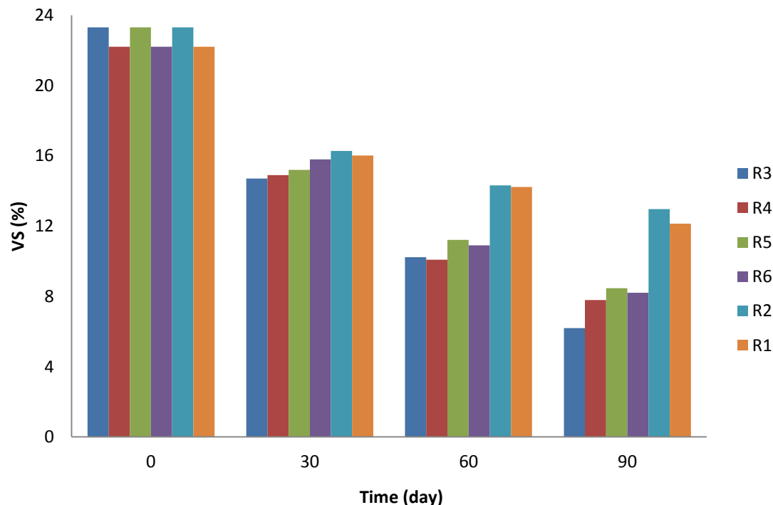
شکل ۳: روند تغییرات VS در راکتورهای مختلف طی فرآیند کمپوست (۹۰ روز)
