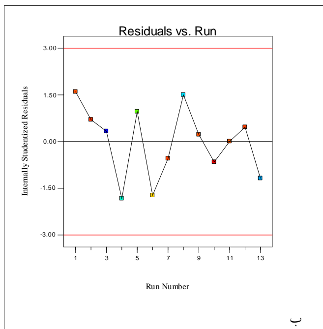
نمودار ۴: پراکنش باقیمانده‌ها نسبت به ترتیب انجام آزمایش‌های غیرفعال سازی الف: کل کلی فرم‌ها و ب: کلی فرم‌های مدفوعی
