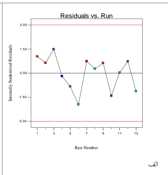
نمودار ۴: پراکنش باقیمانده‌ها نسبت به ترتیب انجام آزمایش‌های غیرفعال سازی الف: کل کلی فرم‌ها و ب: کلی فرم‌های مدفوعی
