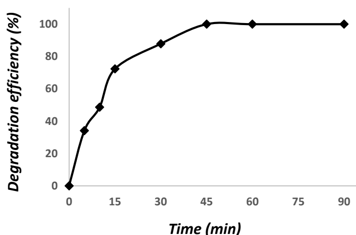
نمودار ۵: تأثیر زمان واکنش بر روی راندمان حذف (۱۰ میلی گرم در لیتر سفنازید، pH=۱۱، دوز کاتالیست ۲ g/L و دوز ازن ۲۲ گرم بر ساعت).
