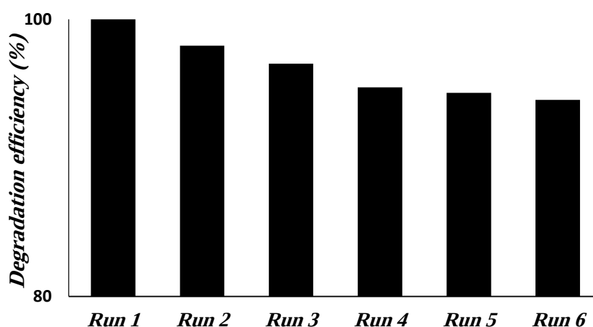
نمودار ۹: بررسی قابلیت استفاده مجدد کاتالیست کاتالیزوری (غلظت سفنازید 10 \text{ mg/l} ، \text{pH}=11 اولیه، دوز کاتالیست 2 \text{ g/L} ، دوز ازن 0.22 \text{ g} بر ساعت)
