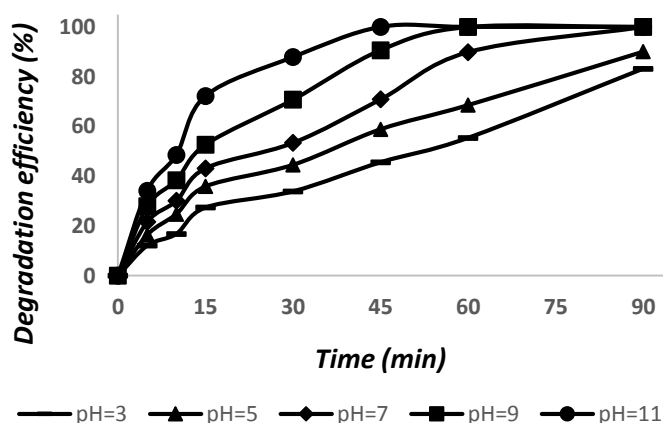
نمودار ۱: تأثیر pH اولیه محلول بر راندمان فرایند (۱۰ میلی گرم در لیتر سفنازید، ۱ گرم در لیتر کاتالیز، دوز ازن ۲۲/۰ گرم بر ساعت).
