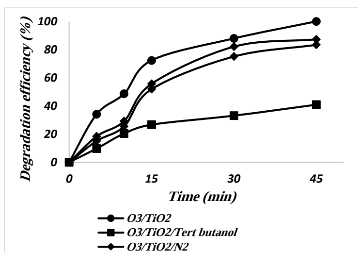
نمودار ۸: بررسی تأثیر بدام انداز رادیکال بر راندمان حذف سفنازید در فرایند ازن زنی کاتالیزوری (غلظت سفنازید 10 \text{ mg/l} ، \text{pH}=11 اولیه، دوز کاتالیست 2 \text{ g/L} ، دوز ازن 0.22 \text{ g} بر ساعت)
