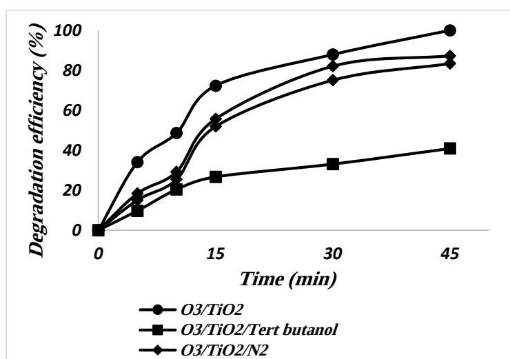
نمودار ۸: بررسی تأثیر بدام انداز رادیکال بر راندمان حذف سفنازید در فرایند ازن زنی کاتالیزوری (غلظت سفنازید 10 \text{ mg/l} ، \text{pH}=11 اولیه، دوز کاتالیست 2 \text{ g/L} ، دوز ازن 0.22 گرم بر ساعت)
