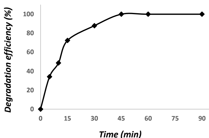
نمودار ۵: تأثیر زمان واکنش بر روی راندمان حذف (۱۰ میلی گرم در لیتر سفتازید، pH=۱۱، دوز کاتالیست ۲ g/L و دوز ازن ۲۲ گرم بر ساعت).
