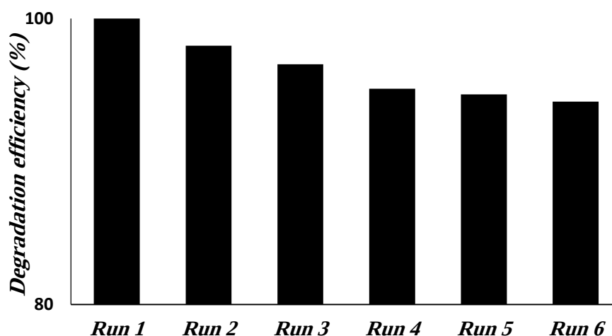
نمودار ۹: بررسی قابلیت استفاده مجدد کاتالیست کاتالیزوری (غلظت سفنازید 10 \text{ mg/l} ، \text{pH}=11 اولیه، دوز کاتالیست 2 \text{ g/L} ، دوز ازن 0.22 گرم بر ساعت)
