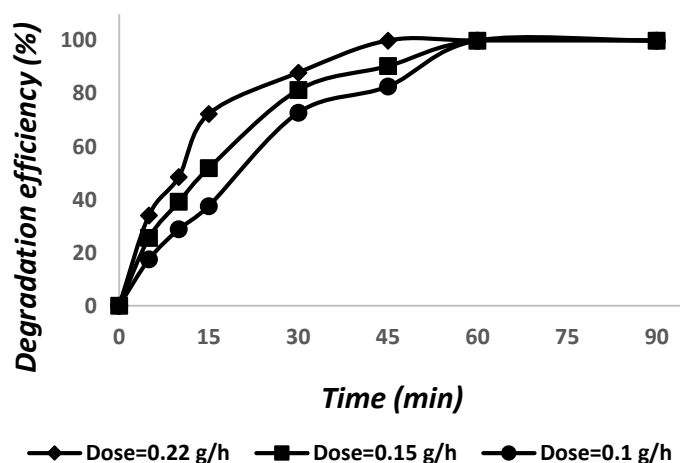
نمودار ۴: تأثیر دوز ازن بر راندمان (pH=۱۱، ۱۰ میلی گرم در لیتر سفتازید)
