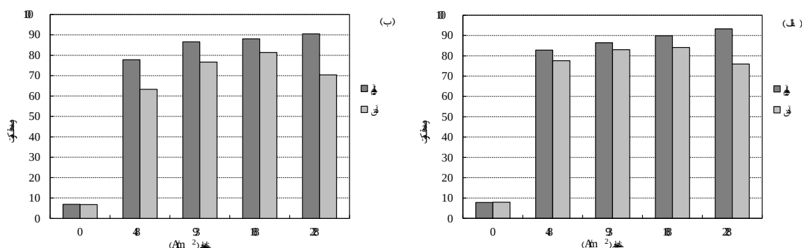
شکل ۸: مقایسه کارایی الکتروالومینیومی و الکترودهنی (سرعت چرخش ۲/۳rpm، زمان ۶۰ دقیقه)، الف: کدورت ۴۲۰ نفلومتری، ب: کدورت ۱۲۰ نفلومتری
