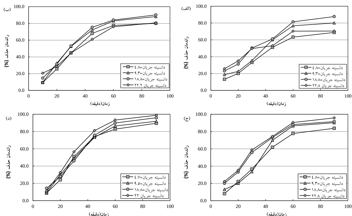
شکل ۴: اثر زمان واکنش و دانسیته جریان بر روی حذف کدورت (سرعت چرخش 2/3 \text{ rpm} ) - (الف: کدورت = 120 نفلومتری، الکتروده آهنی؛ ب: کدورت = 20 نفلومتری، الکتروده آهنی؛ ج: کدورت = 120 نفلومتری، الکتروده آلومینیومی؛ د: کدورت = 20 نفلومتری، الکتروده آلومینیومی)
