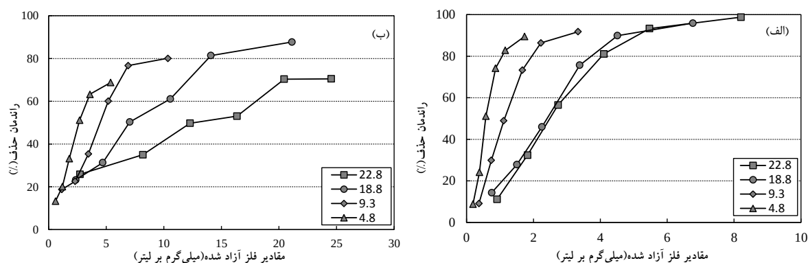
شکل ۶: راندمان حذف کدورت بر اساس مقادیر فلز آزاد شده برای شدت جریان‌های متفاوت (کدورت اولیه ۱۲۰ نفلومتری، سرعت چرخش ۲/۳rpm)، الف: الکترو آلومینیومی، ب: الکترو آهنی
