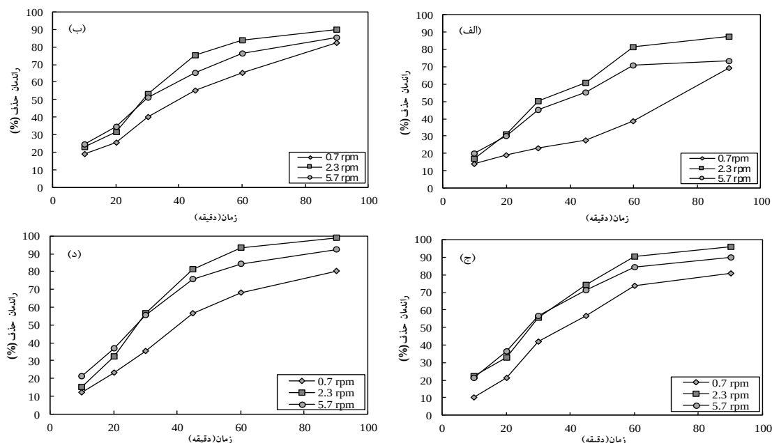
شکل ۳: تغییرات راندمان حذف در مقابل زمان، به ازای سرعت‌های متفاوت چرخش راکتور (دانشیه جریان CD = 18/8 A/m^2 و pH = 7 )، (الف: کدورت=۱۲۰ نفلومتری، الکترود آهنی؛ ب: کدورت=۴۲۰ نفلومتری، الکترود آهنی؛ ج: کدورت=۱۲۰ نفلومتری، الکترود آلومینیومی؛ د: کدورت=۴۲۰، الکترود آلومینیومی)
