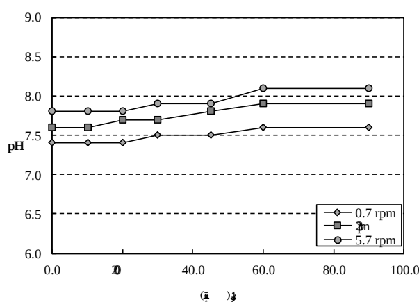
شکل ۹: تغییرات pH با افزایش زمان، الکتروالومینی (کدورت ۲۱۰ نفلومتری، دانسیته جریان ۱۸/۸A/m 2 )
