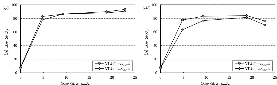
شکل ۵: اثر دانسیته جریان بر روی حذف کدورت (سرعت چرخش ۲/۳rpm، زمان ۶۰ دقیقه)، الف: الکترو د آهنی، ب: الکترو آلومینیومی
