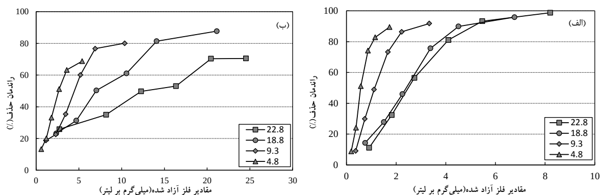
شکل ۶: راندمان حذف کدورت بر اساس مقادیر فلز آزاد شده برای شدت جریان‌های متفاوت (کدورت اولیه ۱۲۰ نفلومتري، سرعت چرخش ۲/۳rpm)، الف: الکترو آلومینیومی، ب: الکترو د آهنی
