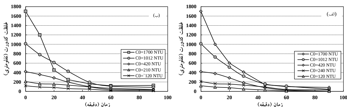
شکل ۷: حذف کدورت در مقابل زمان برای مقادیر غلظت اولیه کدورت متفاوت (دانشیه جریان CD = 18/8A/m^2 ، سرعت چرخش 2/3 rpm و 7/4 pH=، الف: الکتروالومینیومی ب: الکتروالونی)
