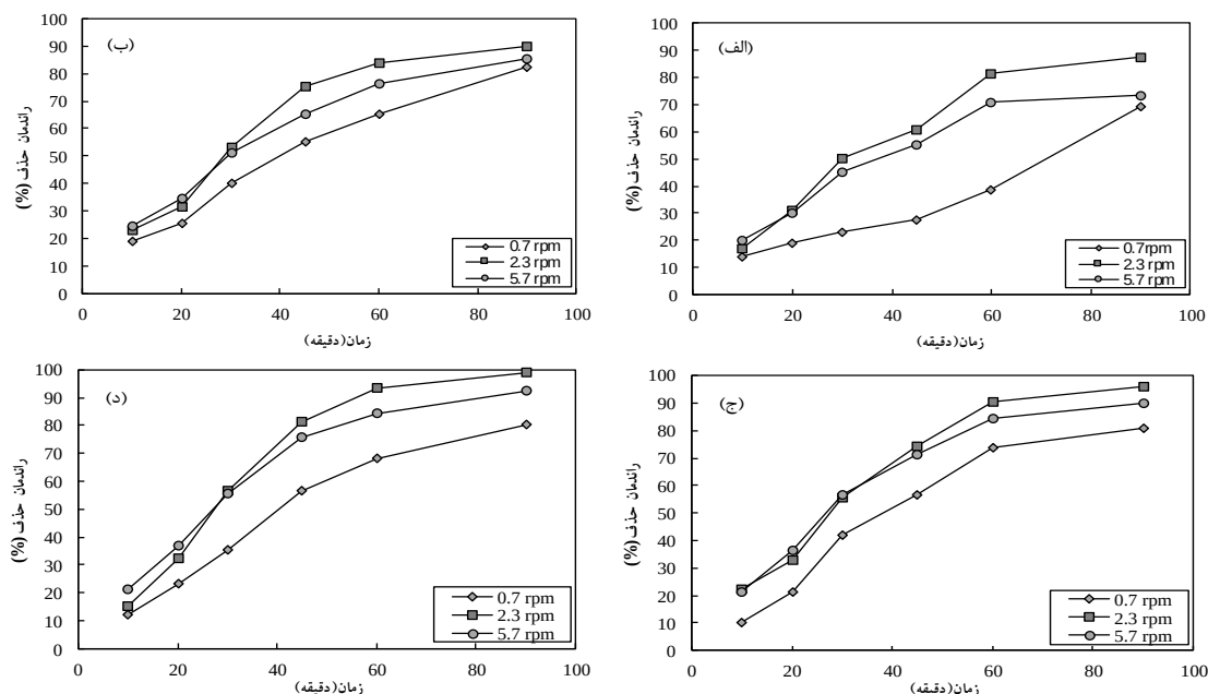
شکل ۳: تغییرات راندمان حذف در مقابل زمان، به ازای سرعت‌های متفاوت چرخش راکتور (دانسیته جریان CD = 18/8 A/m^2 و pH=7 ، (الف: کدورت=۱۲۰ نفلومتری، الکترود آهنی؛ ب: کدورت=۴۲۰ نفلومتری، الکترود آهنی؛ ج: کدورت=۱۲۰ نفلومتری، الکترود آلومینیومی؛ د: کدورت=۴۲۰، الکترود آلومینیومی)
