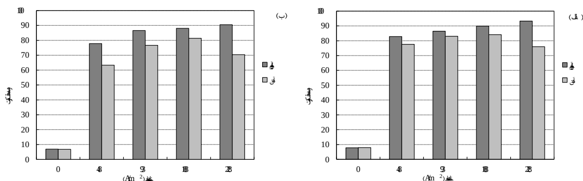
شکل ۸: مقایسه کارایی الکتروالومینیوم و الکتروالومینیوم (سرعت چرخش ۲/۳rpm، زمان ۶۰ دقیقه)، الف: کدورت ۴۲۰ نفلومتری، ب: کدورت ۱۲۰ نفلومتری
