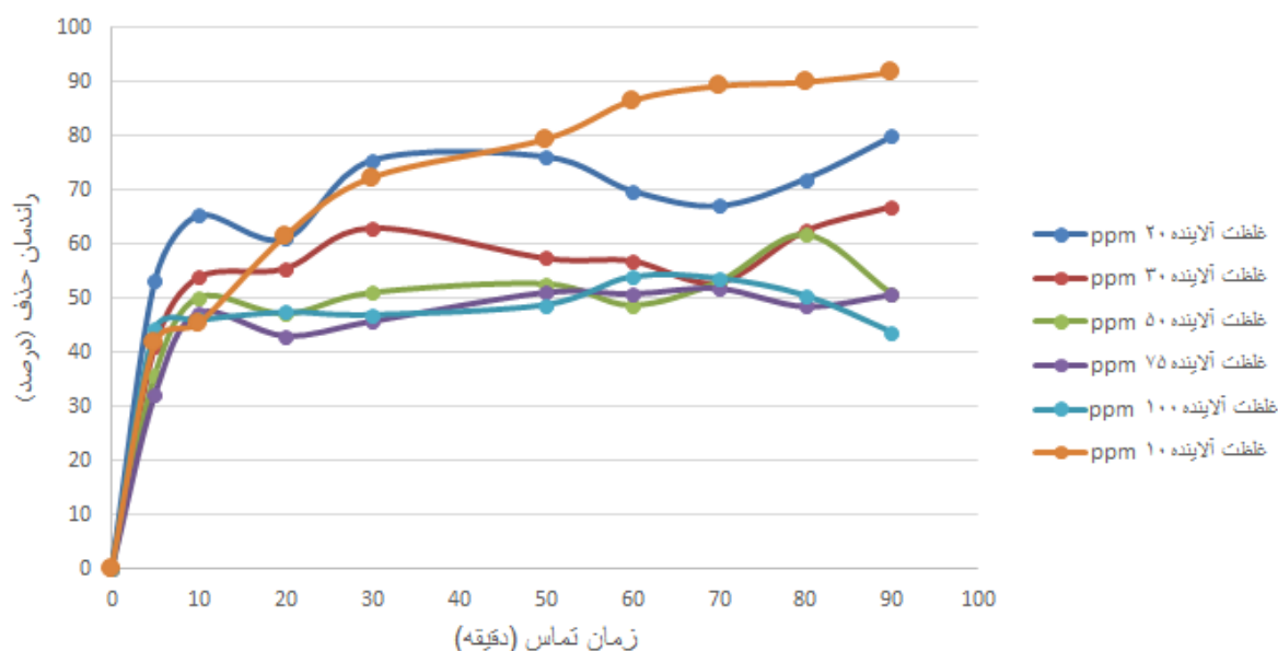
شکل ۷. راندمان حذف آلایندہ آنیلین توسط نانو لوله کربن مغناطیسی شده از محلول با تاثیر غلظت های مختلف آلایندہ آبی با تاثیر pH
