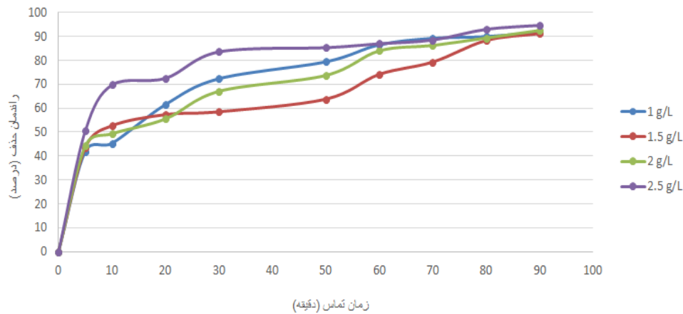
شکل ۶. راندمان حذف آلایندہ آنیلین توسط نانو لوله کربن مغناطیسی شدہ از محلول با تاثیر غلظت های مختلف جاذب
