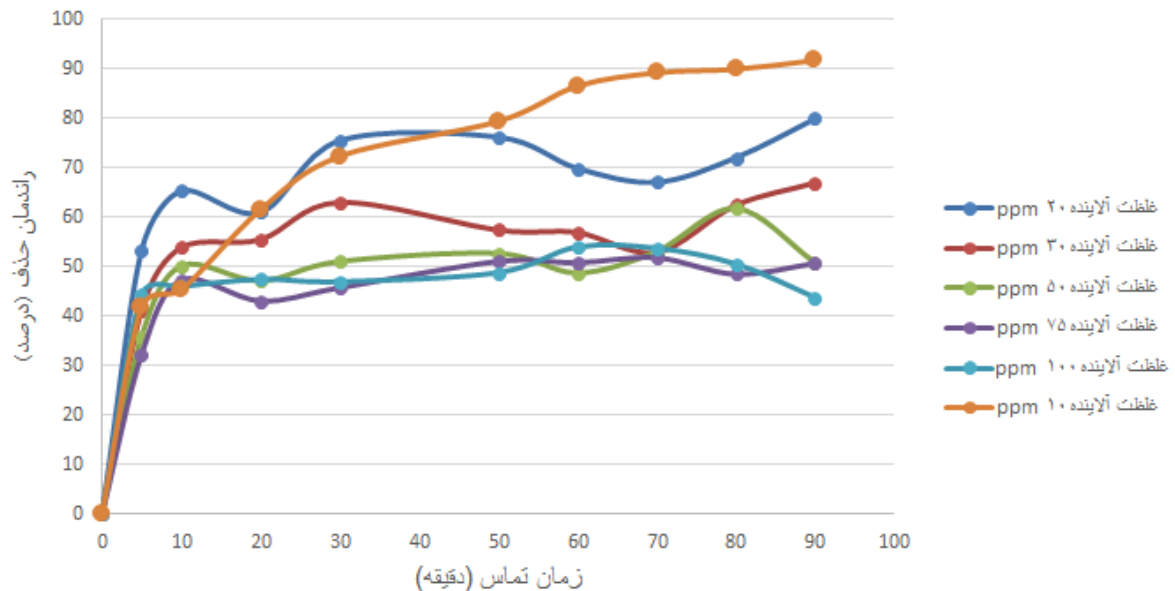
شکل ۷. راندمان حذف آلایندہ آنیلین توسط نانو لوله کربن مغناطیسی شدہ از محلول با تاثیر غلظت های مختلف آلایندہ آبی با تاثیر pH
