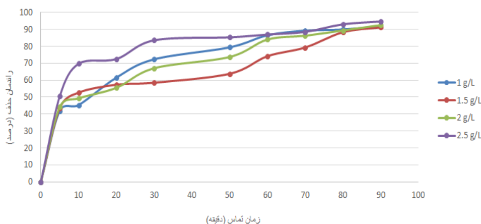
شکل ۶. راندمان حذف آلایندہ آنیلین توسط نانو لوله کربن مغناطیسی شده از محلول با تاثیر غلظت های مختلف جاذب
