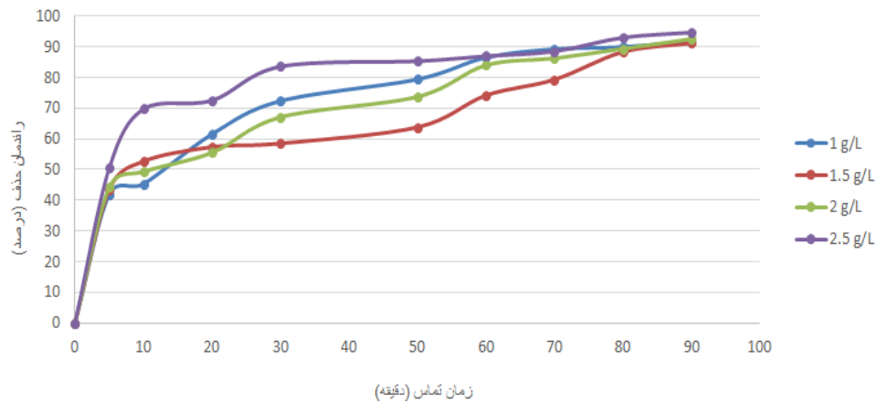
شکل ۶. راندمان حذف آلایندہ آنیلین توسط نانو لوله کربن مغناطیسی شده از محلول با تاثیر غلظت های مختلف جاذب
