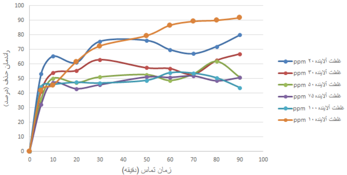
شکل ۷. راندمان حذف آلایندہ آنیلین توسط نانو لوله کربن مغناطیسی شده از محلول با تاثیر غلظت های مختلف آلایندہ آبی با تاثیر pH
