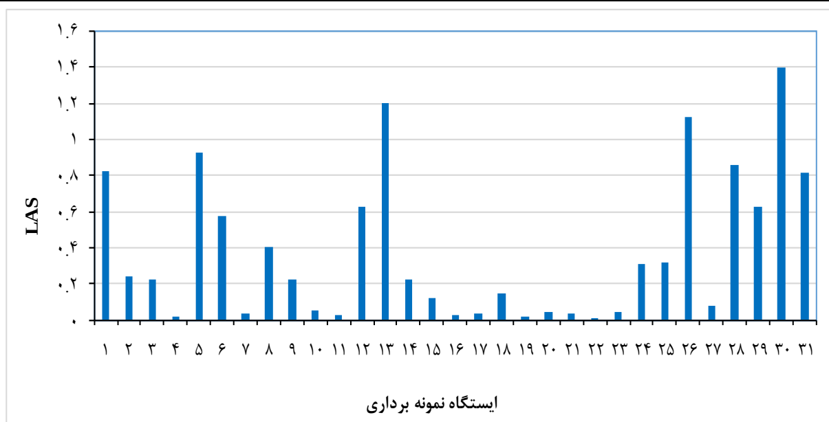
نمودار ۱: غلظت LAS در ایستگاه‌های مورد مطالعه در نمونه آب سد اکباتان
