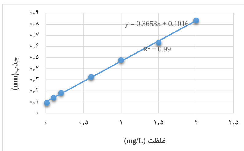
شکل ۲: منحنی کالیبراسیون آلکیل بنزن سولفونات خطی در غلظت‌های مختلف
