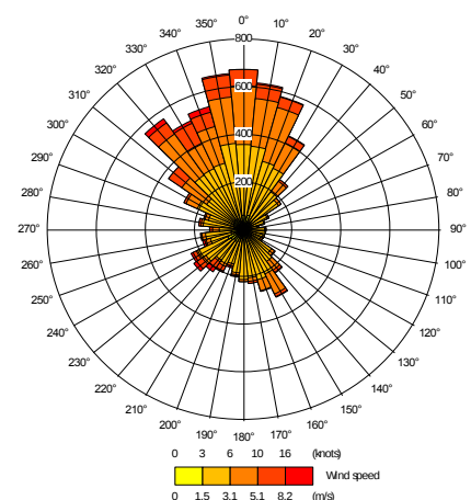
شکل ۸: گلباد منطقه مورد مطالعه
