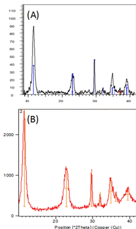
شکل ۱: الگوی پراش اشعه ایکس ماده هیدروکسید لایه‌ای آلومینیوم-منیزیم (A) قبل و (B) از جذب یون کلرید
