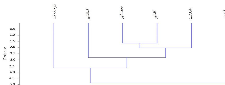
شکل ۴: دندروگرام حاصل از آنالیز خوشه‌ای متغیرهای مورد بررسی در نهشت اتمسفری منطقه مطالعاتی کرج
