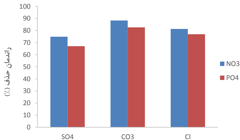
شکل ۷: تأثیر آنیونهای مزاحم بر راندمان حذف نیترات و فسفات توسط جاذب کیتوزان مغناطیسی شده بی متالیک
