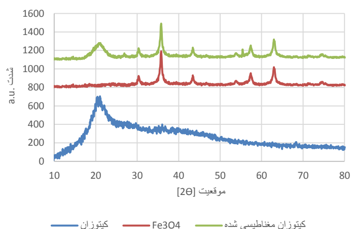
شکل ۲: پراش اشعه ایکس برای کیتوزان و کیتوزان مغناطیسی شده در محدوده زاویه 2\theta = 10^\circ تا 80^\circ
