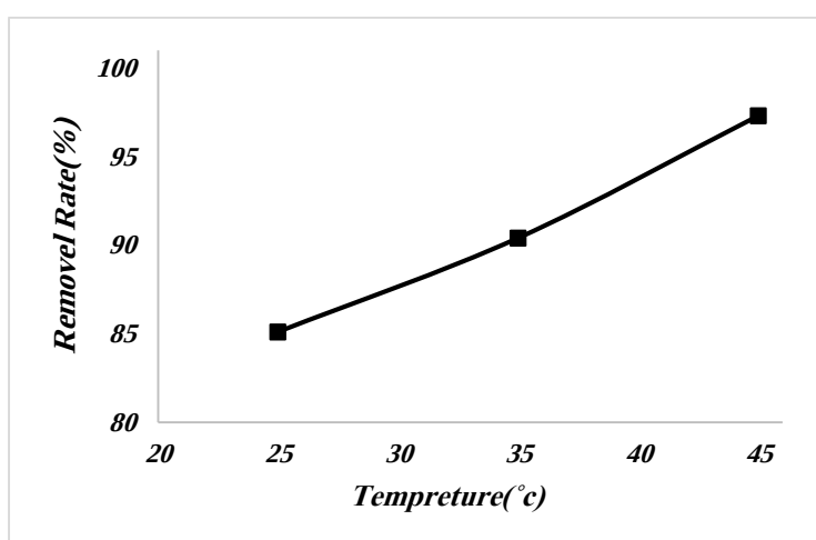
شکل ۶: تأثیر دما بر کارایی جذب جیوه با استفاده از MBSA (غلظت اولیه جیوه ۵۰۰ \mu\text{g/L} ، pH = ۵، زمان تماس برابر ۸۰ دقیقه و دوز جاذب ۰/۲ g/L)
