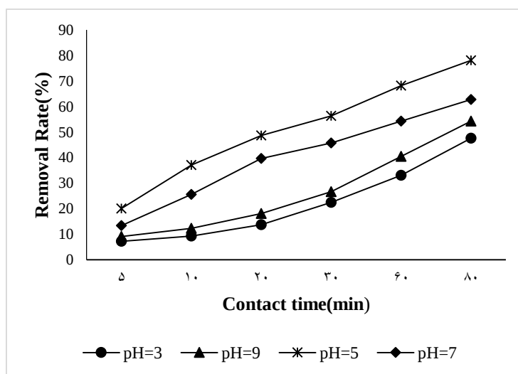
شكل ٣: نتايج مربوط به تاثير pH اوليه بر كارايي حذف جيوه با استفاده از MBSA (غلظت اوليه جيوه ٥٠٠ ميكروگرم بر ليتر، دوز جاذب ٠/١ گرم بر ليتر، دماي ٢٥ درجه سلسيوس)
