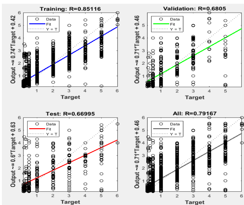
شکل ۸: مقایسه مقادیر متناظر مشاهداتی و محاسباتی با شبکه عصبی دوم برای مراحل آموزش، ارزیابی و آزمون
