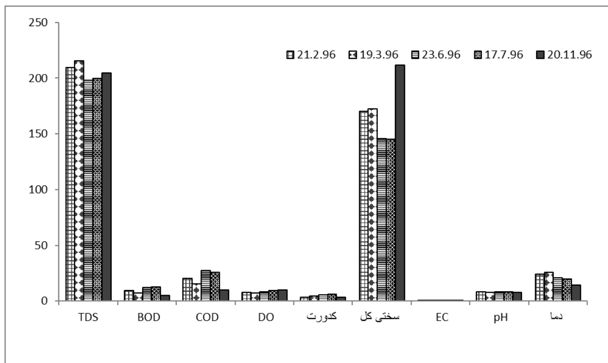
شکل ۳: مقایسه میانگین پارامترهای فیزیکی و شیمیایی اندازه گیری شده نمونه‌های آب در زمان‌های مختلف (پارامترهای TDS, BOD, COD, DO و سختی کل بر اساس میلی گرم بر لیتر، کدورت بر اساس NTU، EC بر اساس دسی زیمنس بر متر و دما بر اساس درجه سانتی گراد بیان شده اند)
