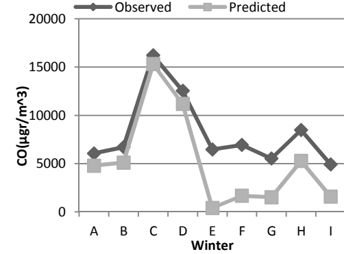
شکل ۳: مقایسه مقادیر شبیه‌سازی و پای‌CO در ۹ ایستگاه پذیرنده
