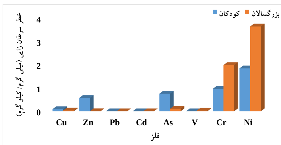
شکل ۴: خطر سرطان‌زایی فلزات سنگین خاک سطحی منطقه صنعتی ماهشهر به تفکیک بزرگسالان و کودکان.
