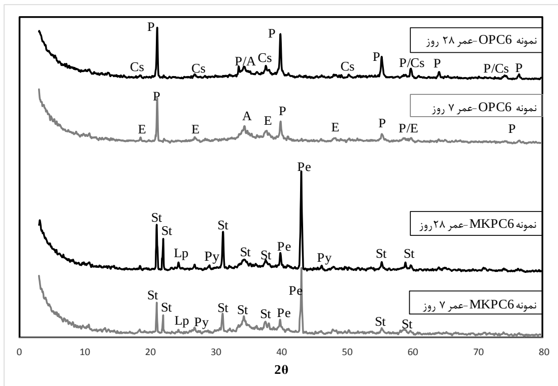
شکل ۴: الگوریتم XRD نمونه‌های ۷ و ۲۸ روزه OPC6 و MKPC6 (St: استرویت - K, Lp: فسفات سرب, Py: پیرومورفیت, Pe: پرکلاس, E: اترینگیت, P: پرتلندیت, A: آلیت Cs: سیلیکات کلسیم هیدراته)
